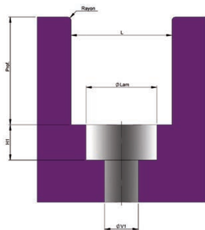
Gorge pour écrou ou grippsters
