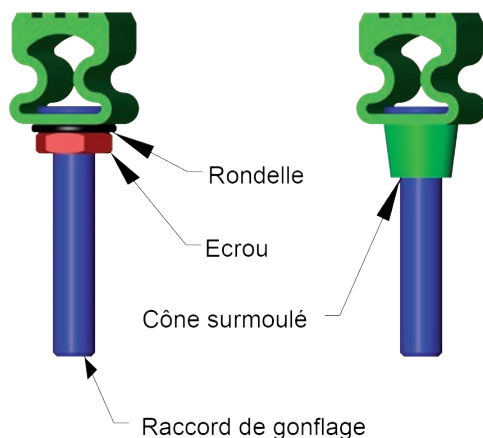
Raccord mécanique
